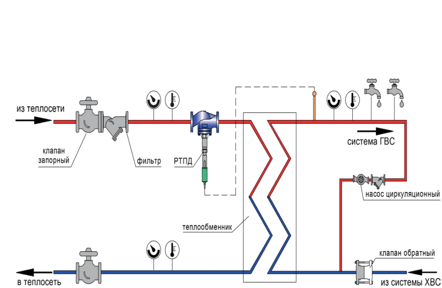
Рисунок 4 – Схема установки РТПД в открытой системе (ГВС)
